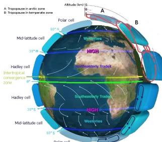
Schematische voorstelling van de afwijking van de dominante windrichting in verschillende circulatiecellen door aardrotatie. Bron: DWindrim via Wikimedia Commons, CC BY-SA 3.0.
